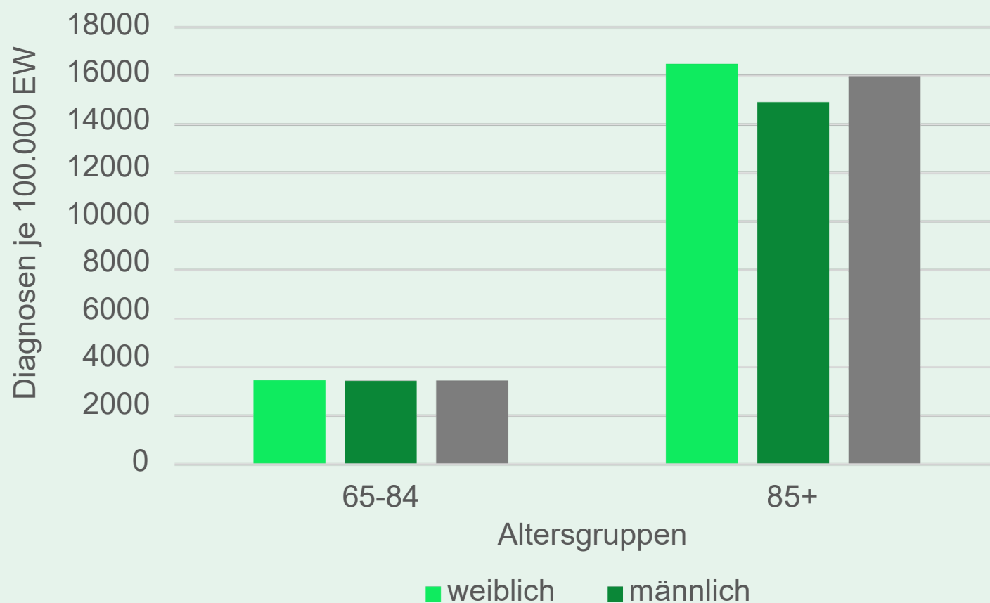
Abb. 2: Häufigkeit von ambulanten Demenzdiagnosen im HSK 2024 nach Altersgruppen (vertragsärztlicher Bereich, je 100.000 Einwohner)
