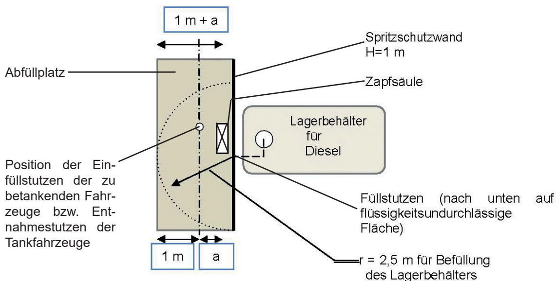
Abbildung 3: Beispiel für die Größe des Abfüllplatzes
