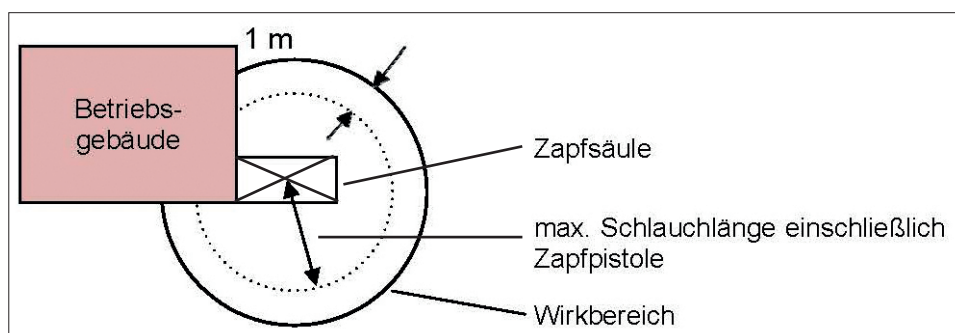
Abbildung 2: Wirkbereich bei der Betankung der Kraftfahrzeuge
